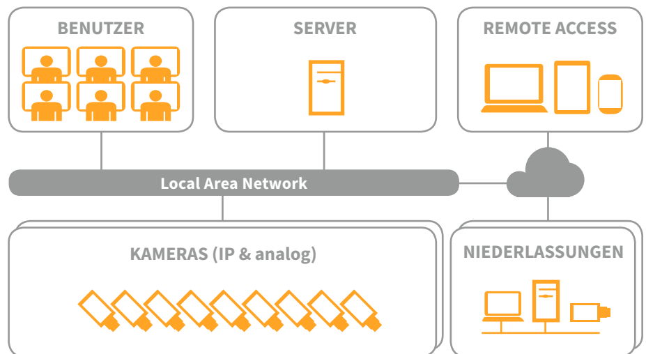
Abbildung: Beispielarchitektur einer Multi-Standort-Installation
